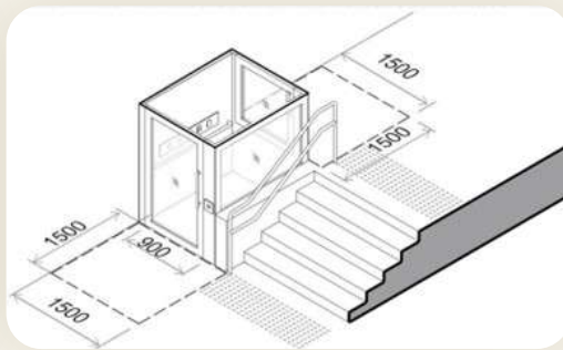
Рисунок 1.42. Приклад влаштування підіймального пристрою з вертикальним переміщенням кабіни.
