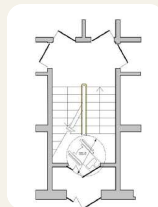
Рисунок 1.34. Схема забезпечення доступності до сходинки на цокольному поверсі
