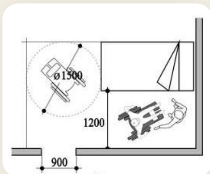
Рисунок 3.16. Схеми убудовування спальні
