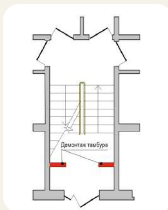
Рисунок 1.34. Схема забезпечення доступності до сходинки на цокольному поверсі
